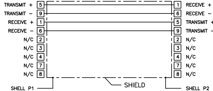
WIRING
